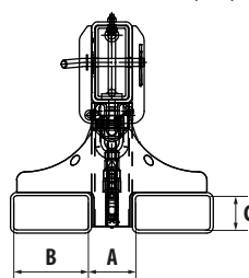
Einfahrtaschen-Innenmaße (mm)
