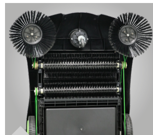
Abb. zeigt HKM 801 mit Tandem-Walzen-System
